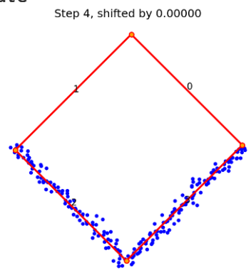
(d) \alpha = 0.20
